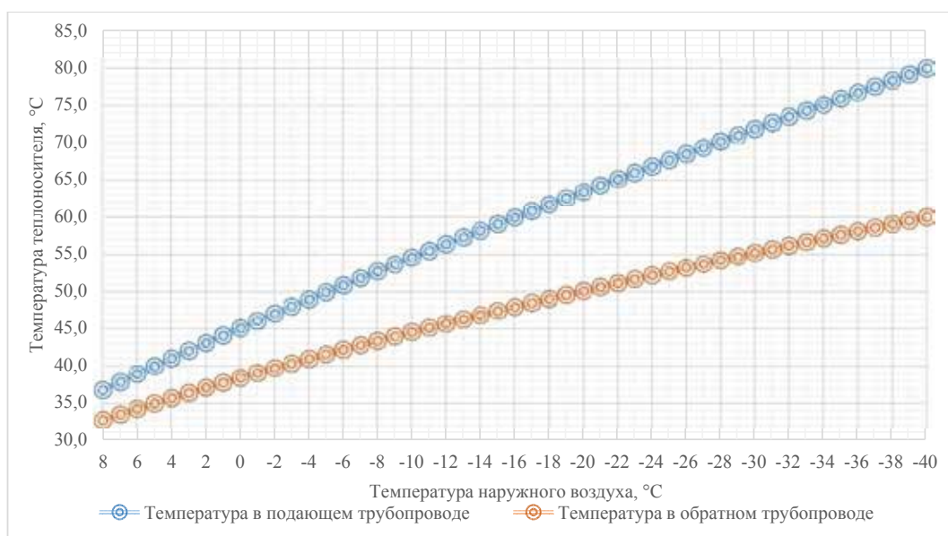
Рисунок *** – Температурный график режима работы котельной «Камышка»
