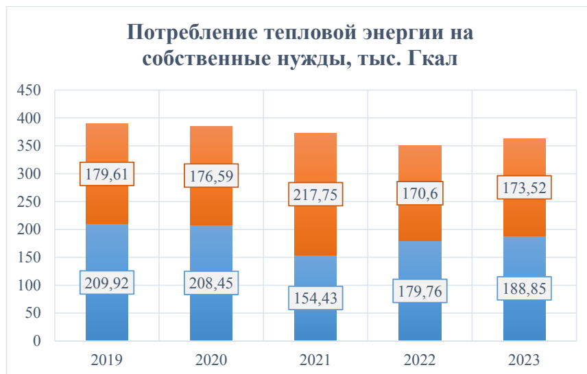
Рисунок *** – Динамика изменения затрат тепловой энергии на собственные нужды ТЭЦ АО «РИР»
