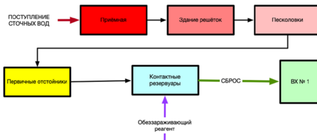
Рисунок *** - Схема КОС г. Северска
