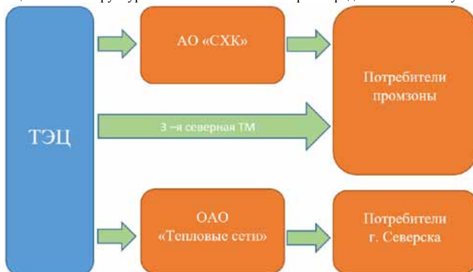
Рисунок *** – Функциональная структура теплоснабжения г. Северска
