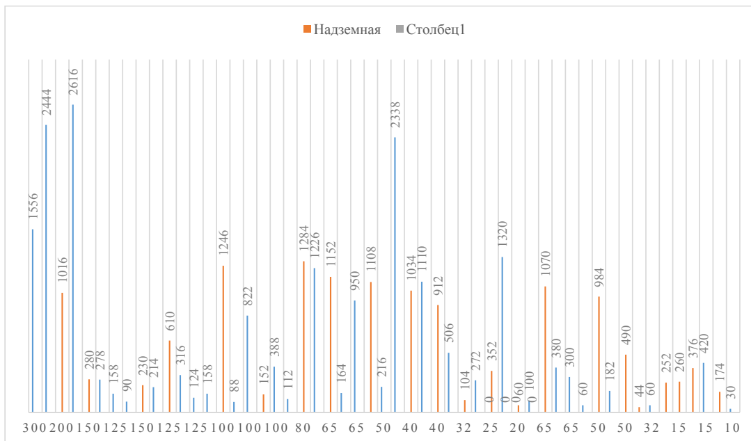
Рисунок *** – Структура тепловых сетей в зоне действия котельной «ЦОК»
