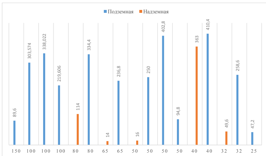
Рисунок *** – Структура тепловых сетей в зоне действия котельной «Камышка»
