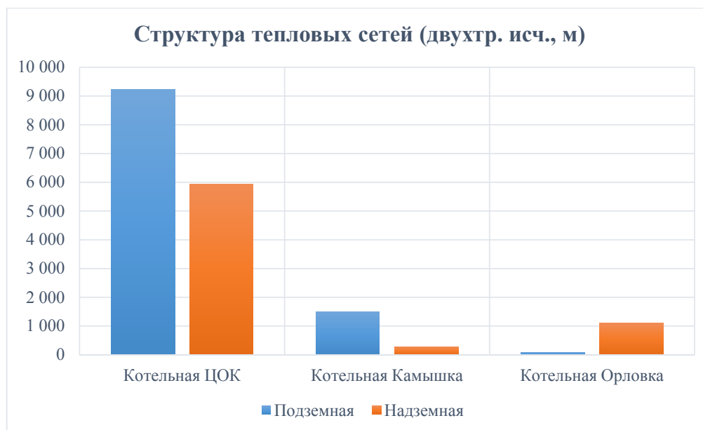
Рисунок *** – Структура тепловых сетей по видам прокладки
