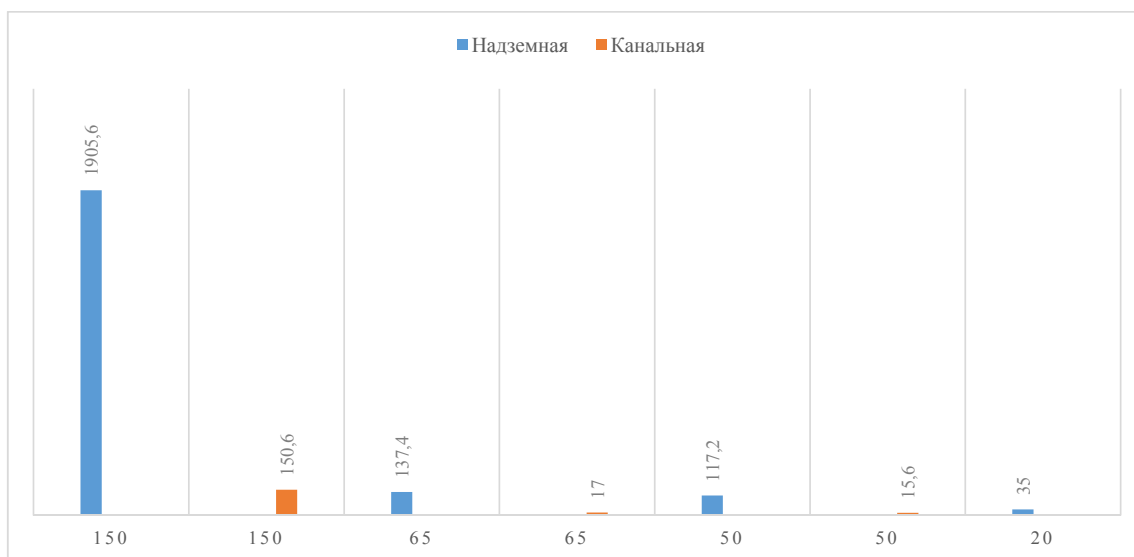
Рисунок *** – Структура тепловых сетей в зоне действия котельной п. Орловка
