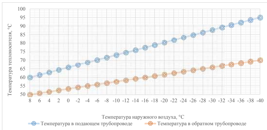
Рисунок *** – Температурный график режима работы котельной «ЦОК»
